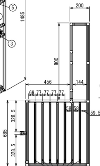
B-B : 3ヶ所 (1 : 15)
