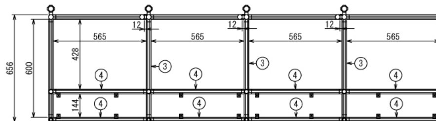
C-C (1 : 15)
