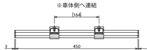
片側の側面図
