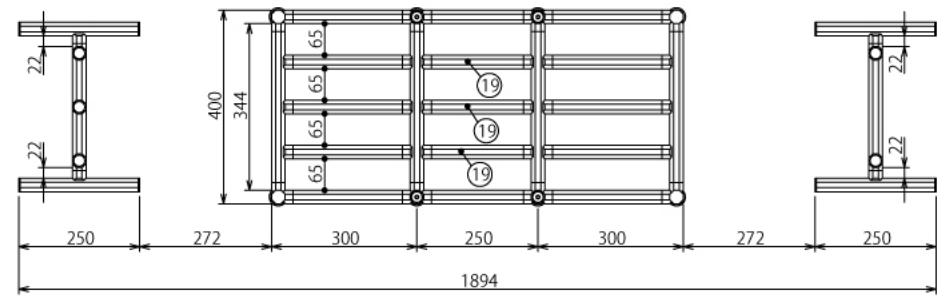
E-E (1 : 10)
