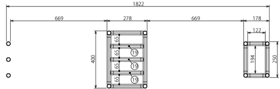
D-D (1 : 10)
