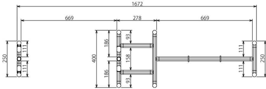
B-B (1 : 10)
