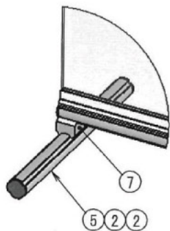
詳細図 B スケール 1:5
