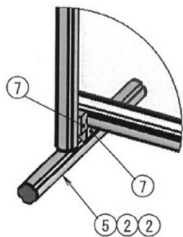
詳細図 B スケール 1 : 5
